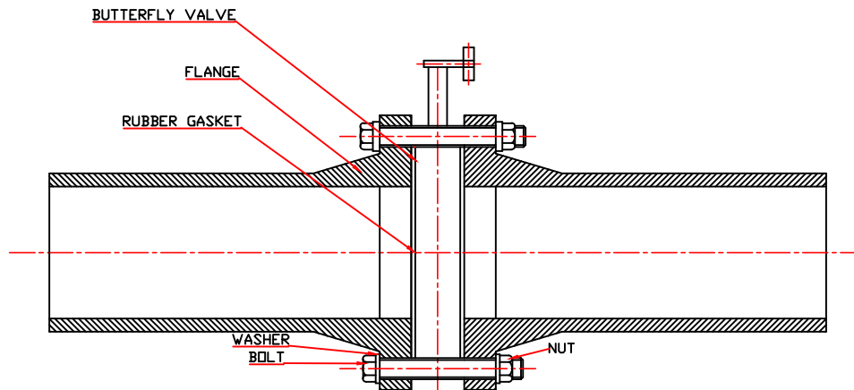
DRG 1.FLANGE
